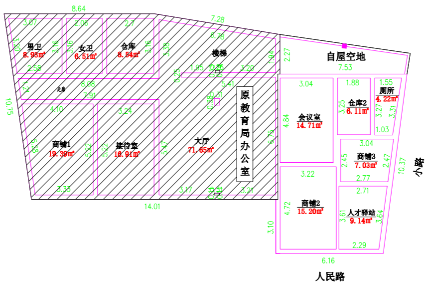
房屋租赁范围平面图（一层） 1:150
